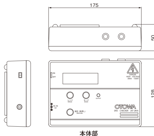
本体部
